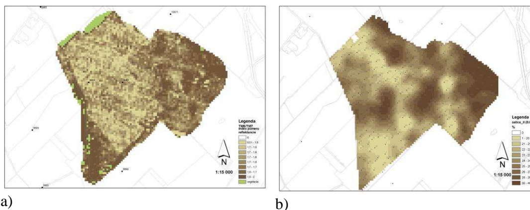
Obr. 3. Výsledok detekcie % obsahu ílu satelitného obrazového záznamu družice Landsat TM ako pomer odrazivosti v hyperspektrálnych oblastiach kanálov TM5/TM7 (3a). Výsledok priestorovej interpolácie (ordinary kriging) pozemných referenčných údajov analytického obsahu frakcie ílu (%) v jemnozemi povrchového A horizontu.
