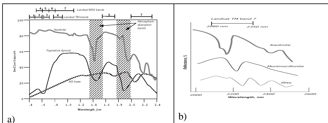
Obr. 2. Spektrálne pásma kanálov TM senzoru družice Landsat s hodnotami odrazivosti vybraných prírodných materiálov (kaolinit, prachovito-hlinitá pôda, vegetácia) (2a) hodnoty odrazivosti kaolinitu, montmorillonitu a illitu v hyperspektrálnom pásme infračervenej oblasti (7 kanál TM senzor) družice Landsat 2.08-2.35µm (2b)
